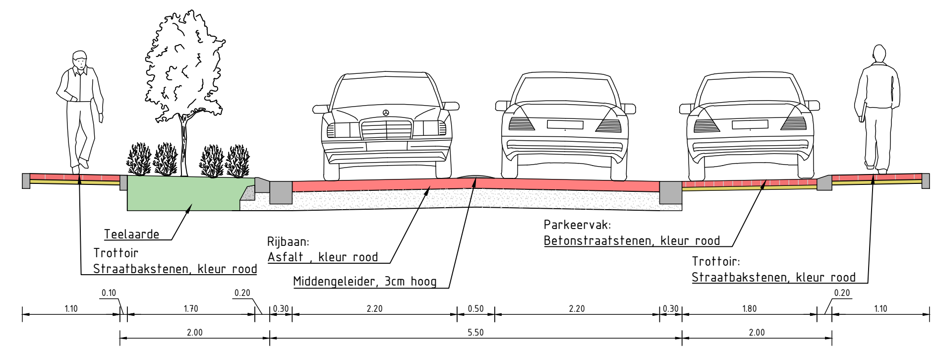
Principe doorsnede (Teelaarde en parkeervak) Schaal 1:50
